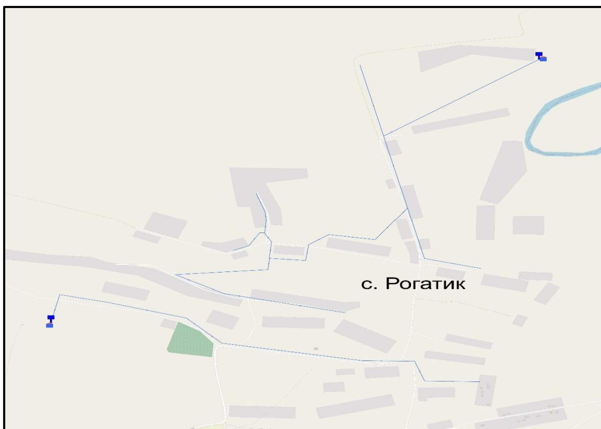
Рис. 2 – Схема водоснабжения с. Рогатик
