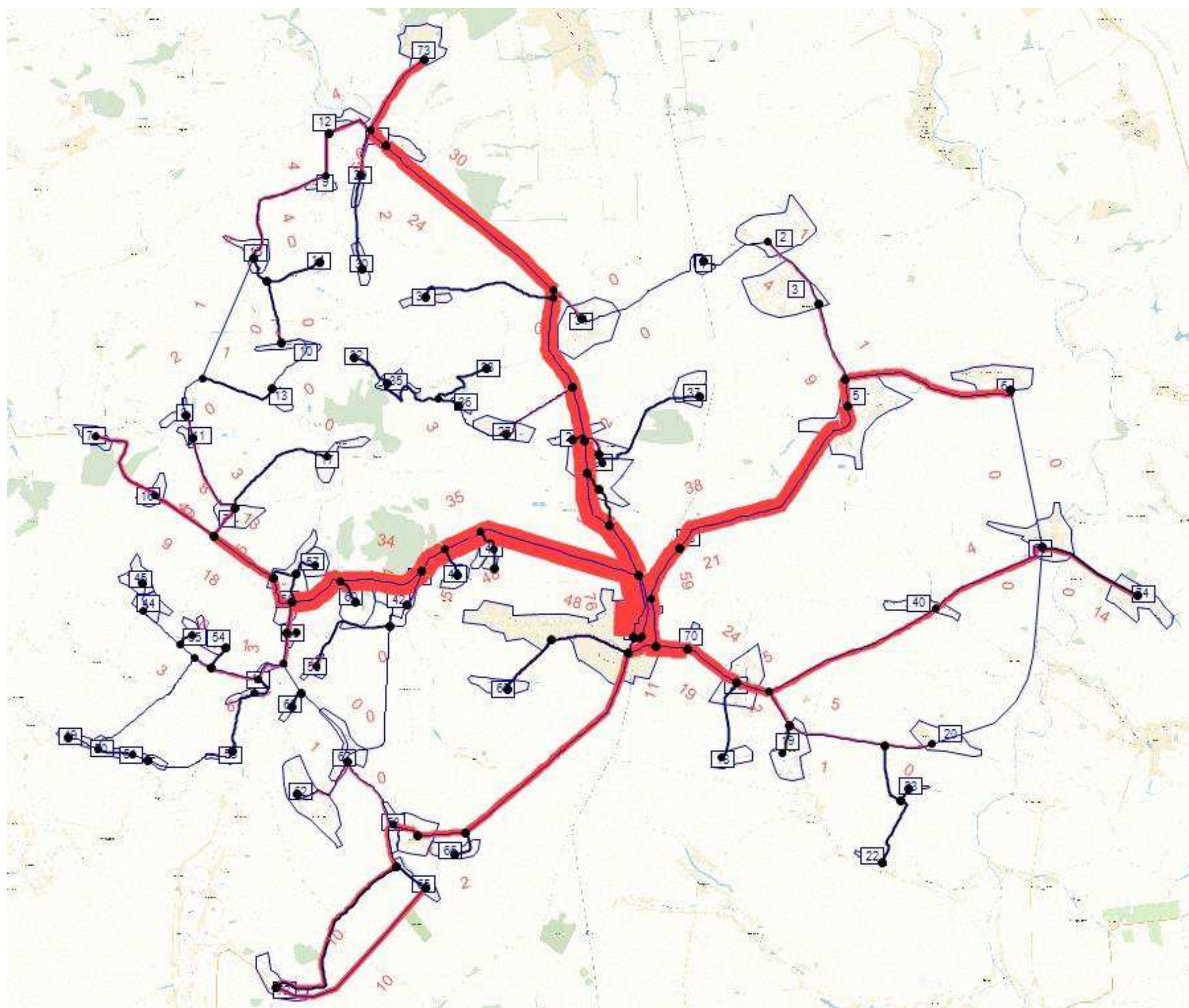
Рассчитанная нагрузка УДС на 2023 год
