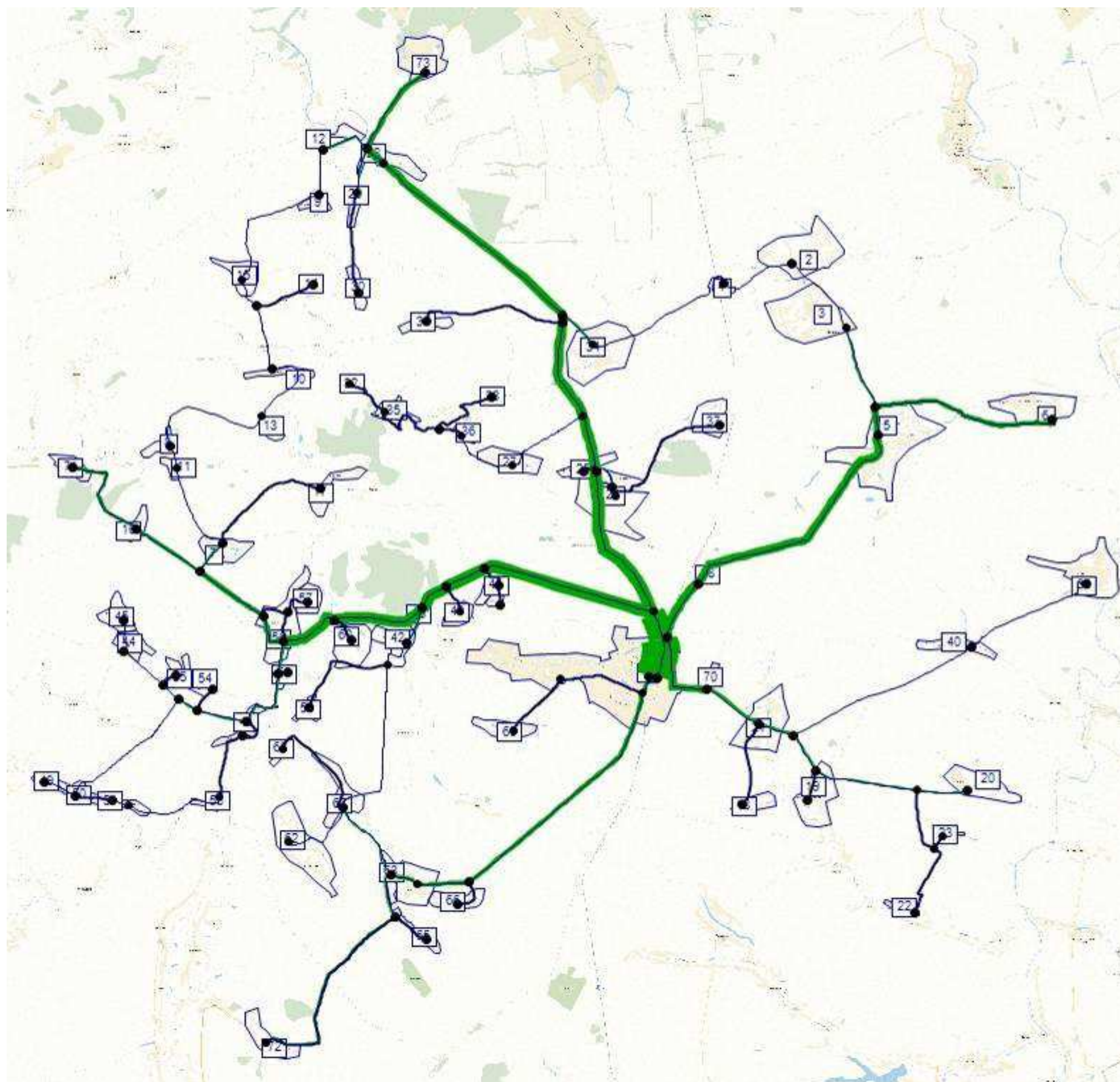
Рассчитанная нагрузка УДС в базовой модели Должанского муниципального района
