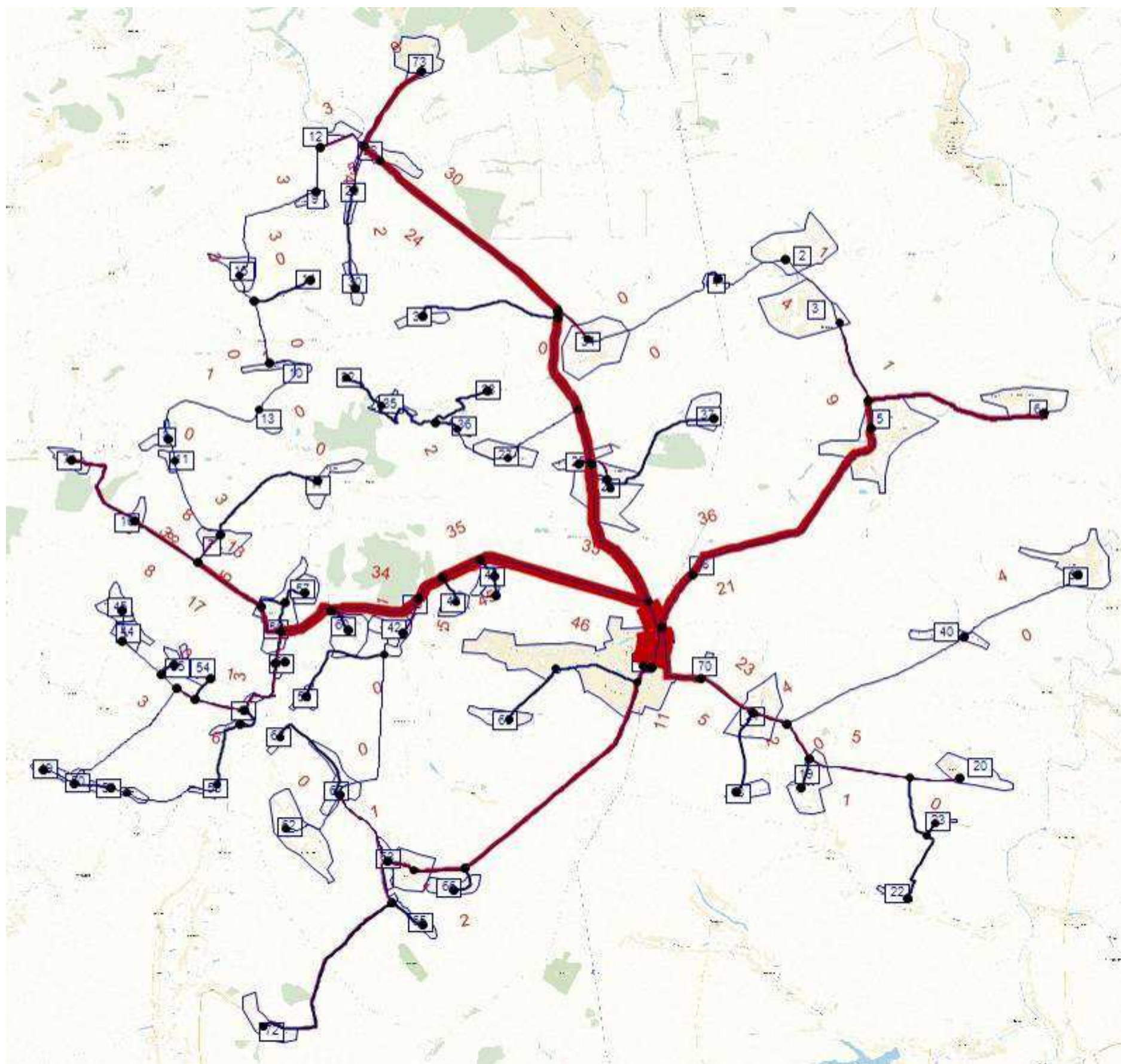
Рассчитанная нагрузка транспорта в базовой модели Должанского муниципального района, в PTV Visum 10
