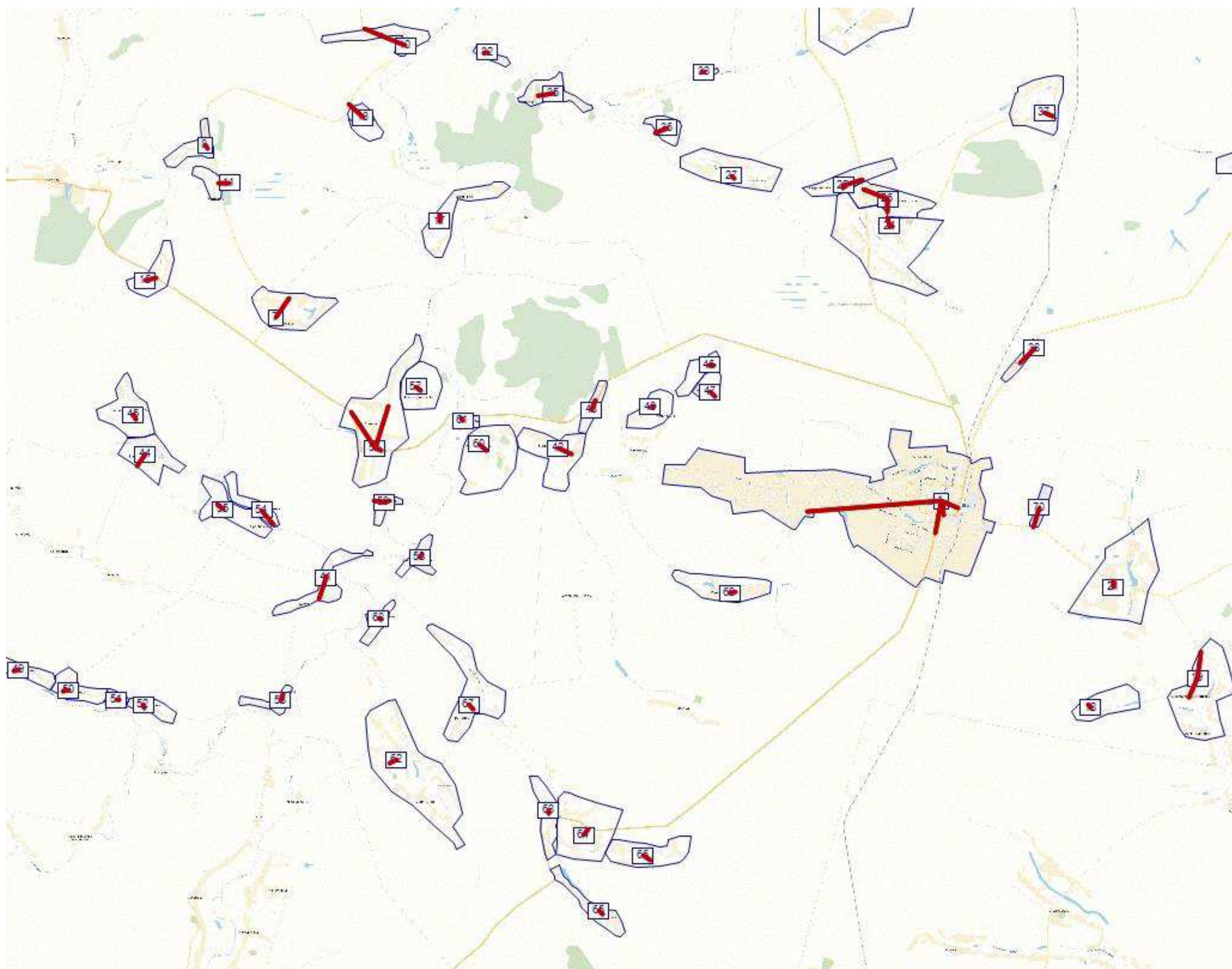
Дуги связи (красным) в модели Должанского района
