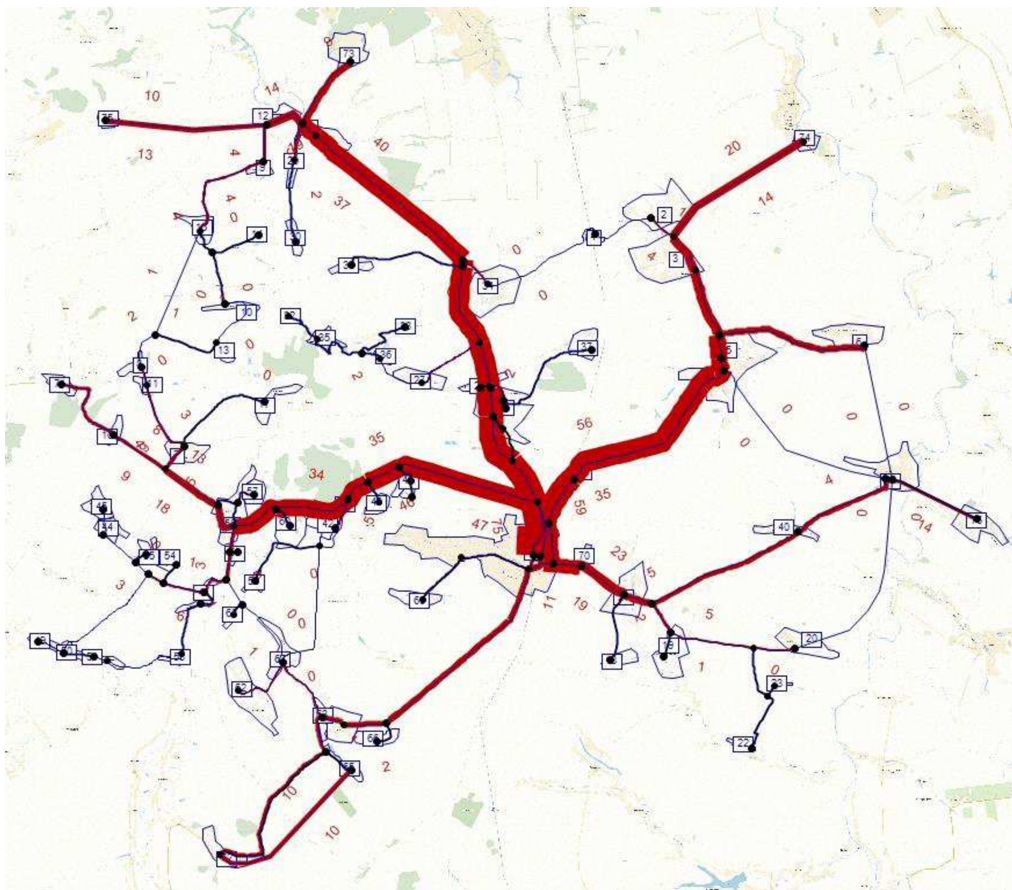
Рассчитанная нагрузка на УДС Должанского муниципального района на перспективу до 2032 года
