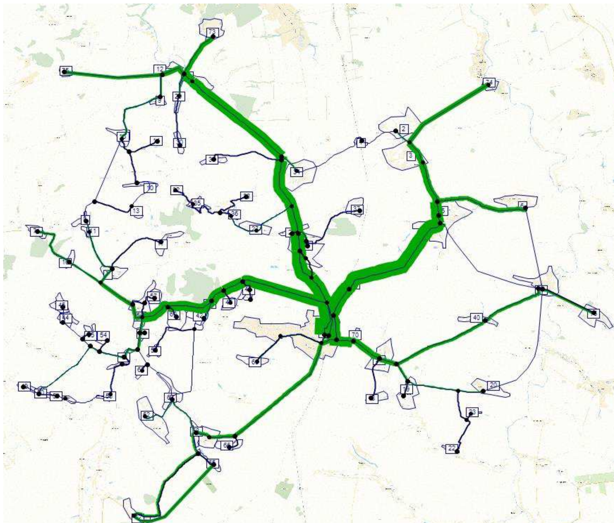
Рассчитанная загрузка УДС Должанского муниципального района на перспективу до 2032 года
