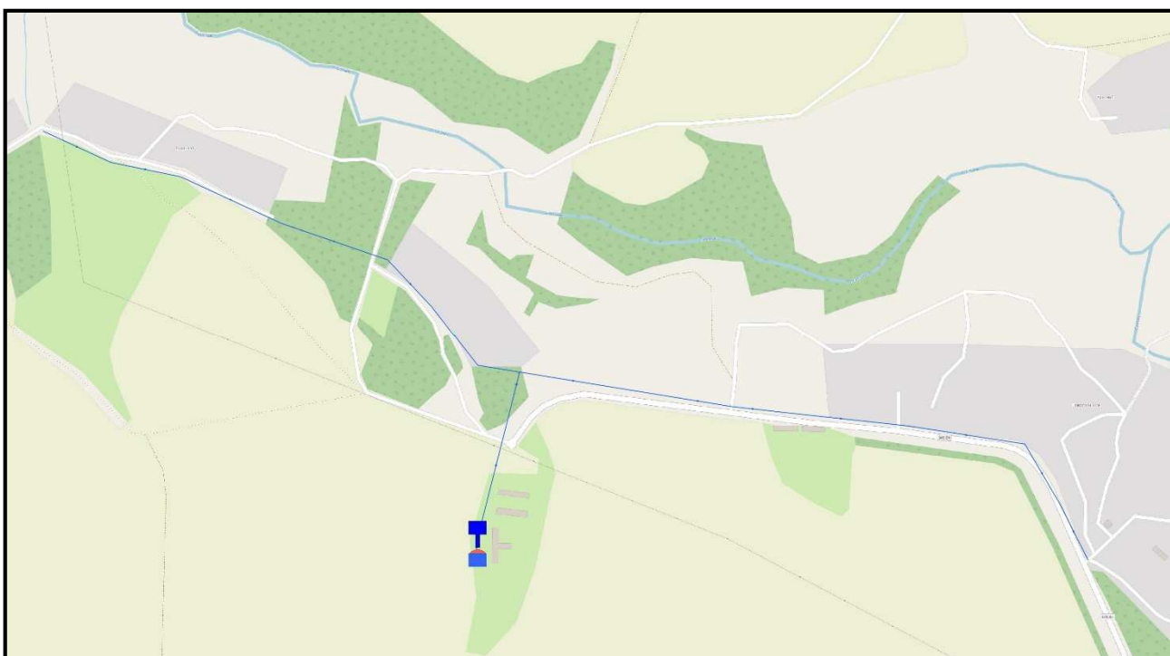
Рис. 4 – Схема водоснабжения п. Кривцова-Плота
