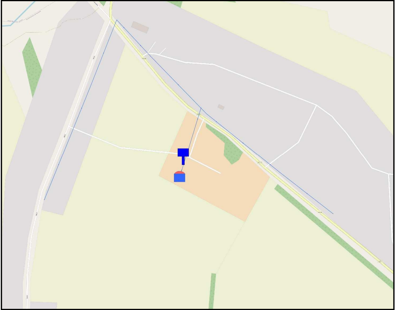
Рис. 2 – Схема водоснабжения д. Евланов, д. Луганка
