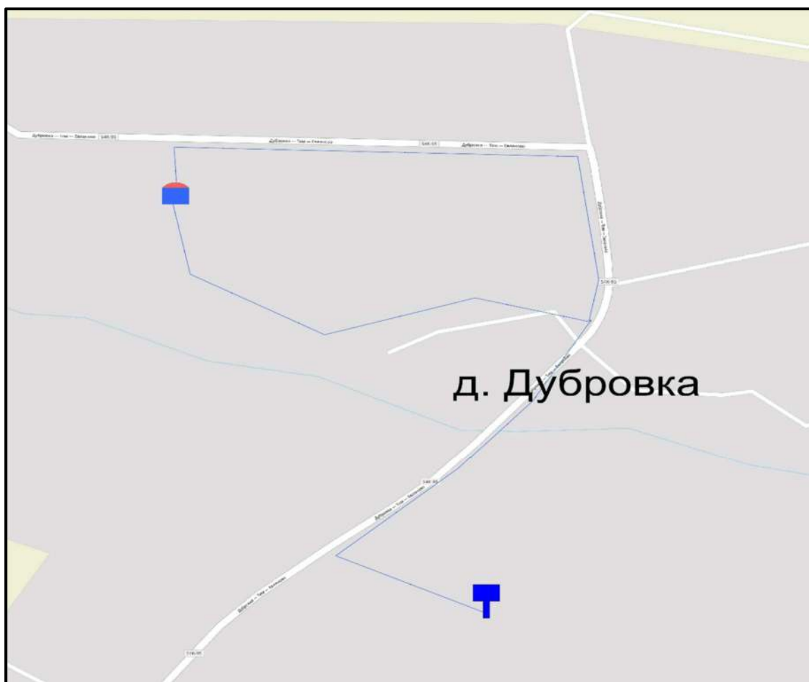
Рис. 2 – Схема водоснабжения д. Дубровка
